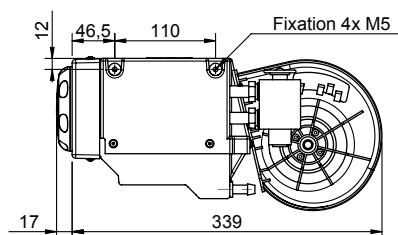
HVAC
