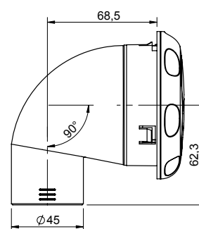
90° D45
